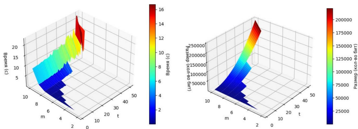
Рис. 2а, 2б. Зависимости времени генерации и размера (соответственно) открытого ключа в зависимости от параметров m и t .
