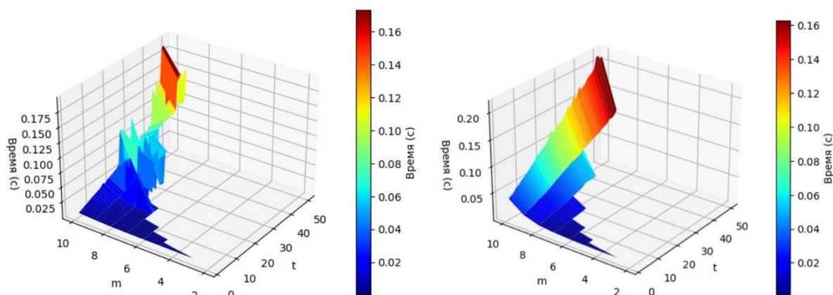
Рис. 3а, 3б. Зависимости времени шифрования и дешифрования (соответственно) в зависимости от параметров m и t .
