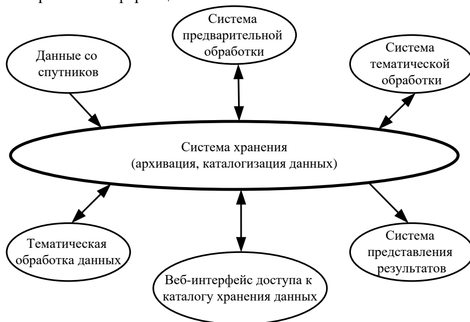
Рис. 1. Структура информационной системы спутникового мониторинга состояния почв.
