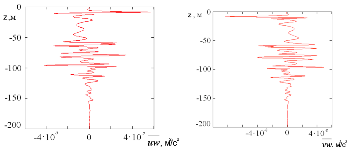
Рис. 1. Профили волновых вертикальных потоков импульсов \overline{uw} и \overline{vw} .
